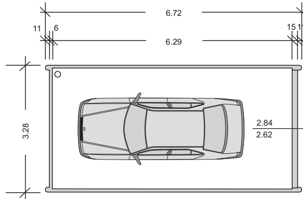
Grundriss Athena B 328 N 262
