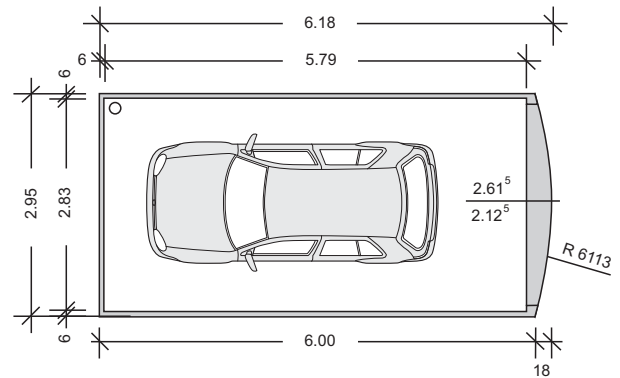
Grundriss Sinus 295 K
